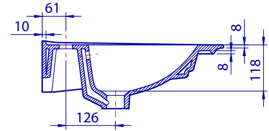
A-A KESİTİ
